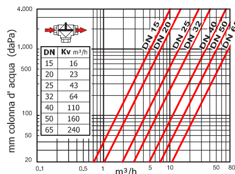
DIAGRAMMA PERDITE DI CARICO
