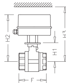
FLANGIA ATTACCO MOTORE ISO 5211
